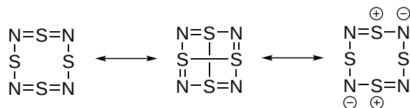
图 17: S_4N_4 的部分共振式示意
