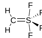
(c) (H_2C)SF_4 的结构
