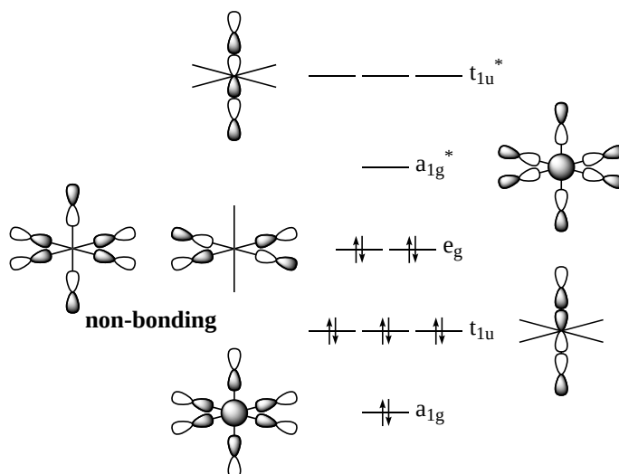
图 14: SF 6 的分子轨道图
